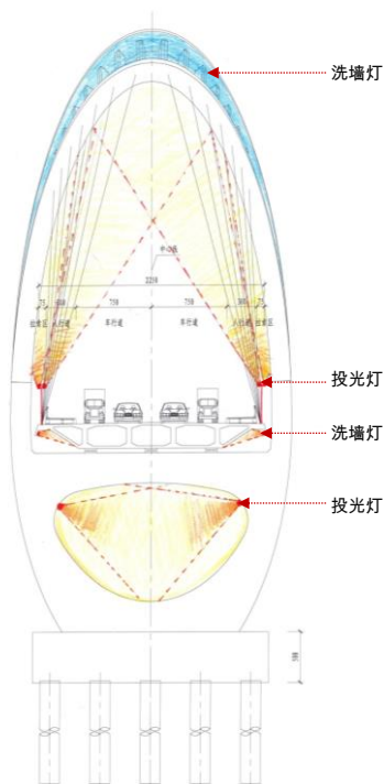
主桥塔剖面图
