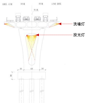
桥墩剖面图
